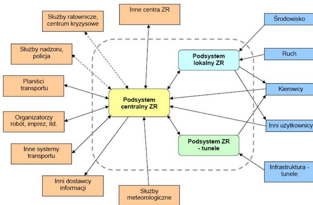
Rys. 3.7 Diagram kontekstowy dla projektowanego SZR
