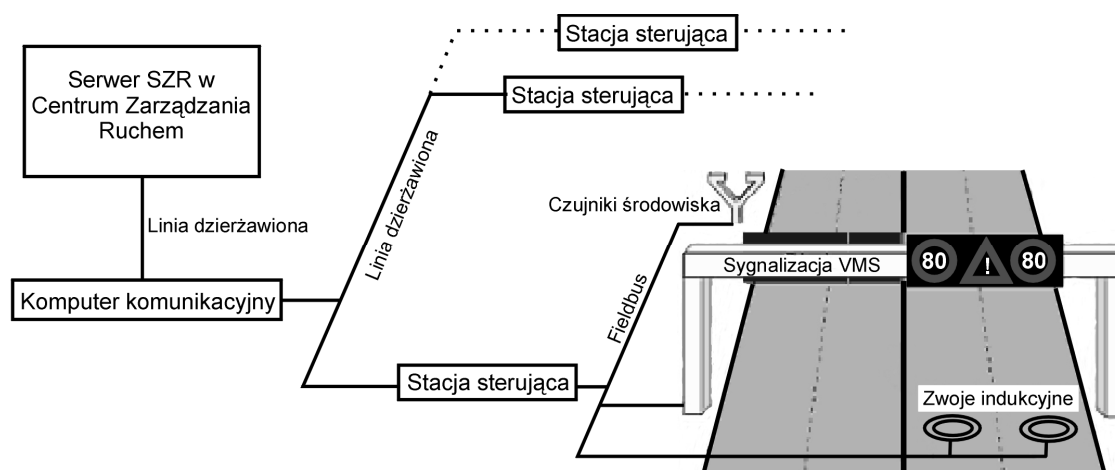
Rys. 2.1: Przykład struktury informatycznej SZR dla autostrad.
