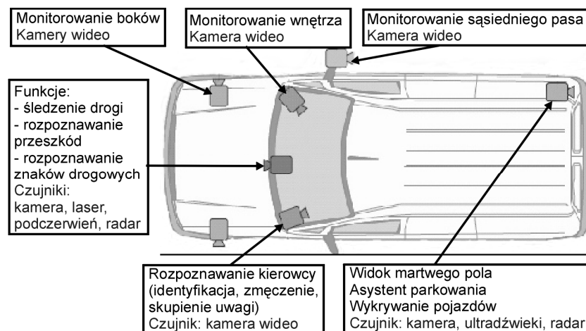
Rys.4.1 Czujniki w pojeździe i ich rola w systemie asystenta kierowcy (według [Broggi 2008])
