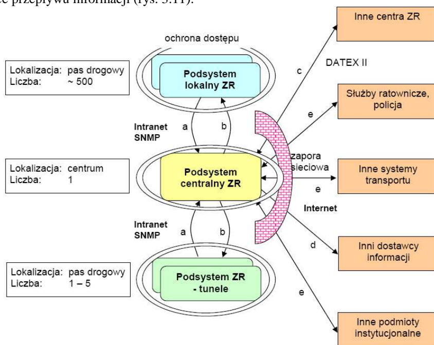
Rys. 3.11 Architektura łączności w systemie SZR.
