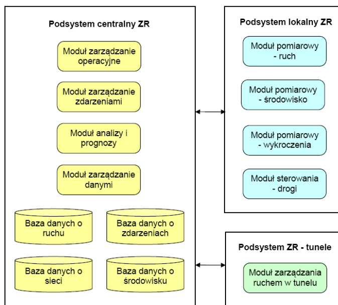
Rys. 3.6: Ilustracja architektury fizycznej dla systemu SZR w WWDK.
