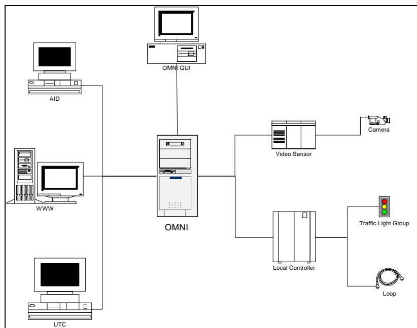
Rys. 2.2: Przykład struktury SZR w ruchu miejskim: (od lewej) aplikacje, centralny serwer (OMNI), sterowniki, czujniki i efekторы [OMNI 2000].
