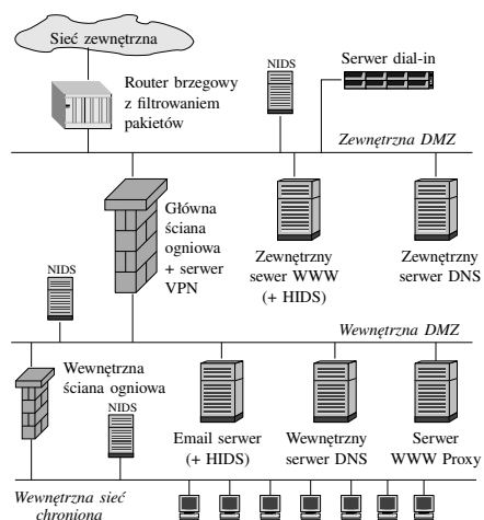
Rysunek 4: Rozbudowana architektura ściany ogniowej.
