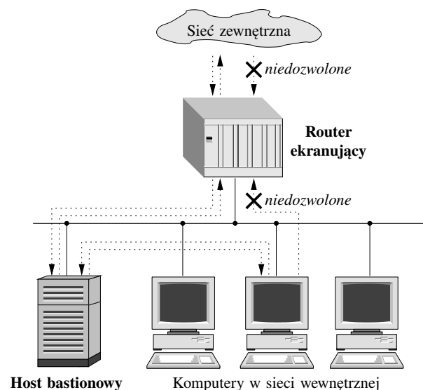
Rysunek 1: Architektura z ekranowanym hostem.
