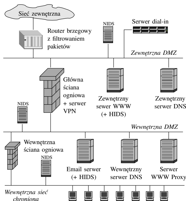
Rysunek 1.4: Rozbudowana architektura ściany ogniowej.
