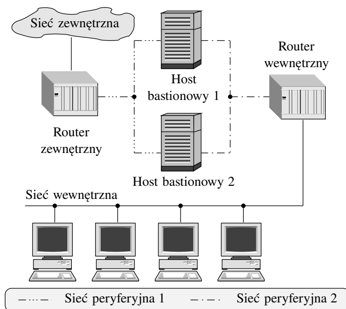
Rysunek 1.3: Architektura dwuczęściowej ekranowanej sieci bez przechodzącego ruchu.
