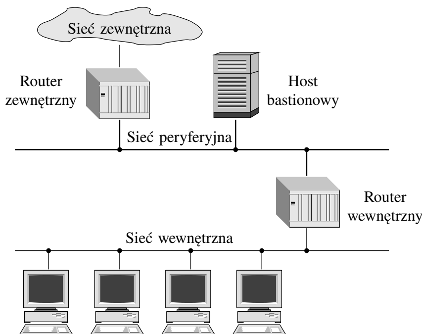
Rysunek 1.2: Architektura ekranowanej podsieci z wykorzystaniem dwóch routerów.
