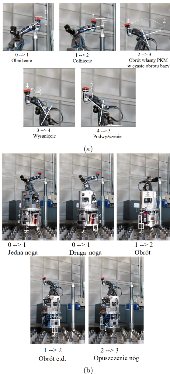
Rys. 6. Ilustracja sekwencji akcji manipulatora i bazy mobilnej dla wykonania pojedynczego przejścia pomiędzy dwoma kolejnymi stanami podparcia blachy przez jednego robota: (a) 5 akcji manipulatora PKM, (b) 3 akcje bazy mobilnej
