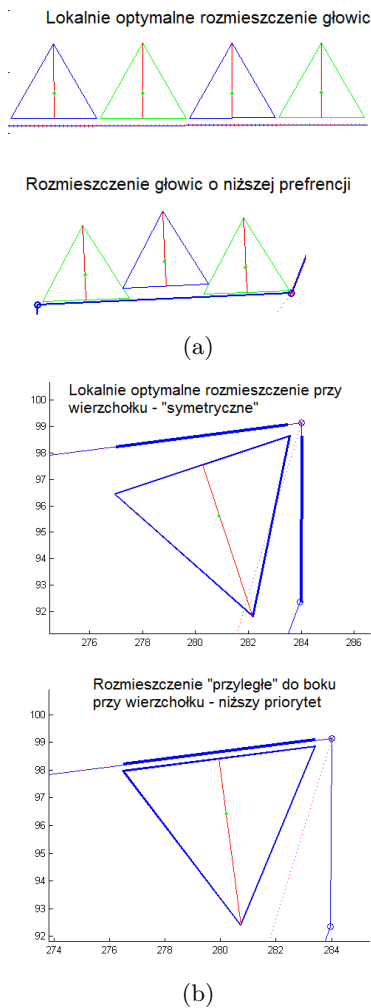
Rys. 4. Ilustracja preferencji rozmieszczania głowic: (a) wzdłuż segmentu liniowego konturu, (b) przy wierzchołku Fig. 4. Illustration of head positioning preferences: (a) at a contour's line segment, (b) at a corner
